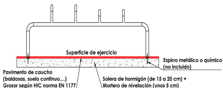
INSTALACIÓN SOBRE SUELO DE HORMIGÓN
