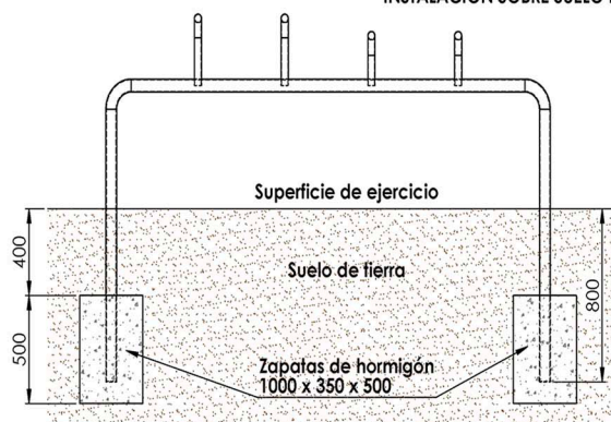
INSTALACIÓN SOBRE SUELO DE TIERRA
