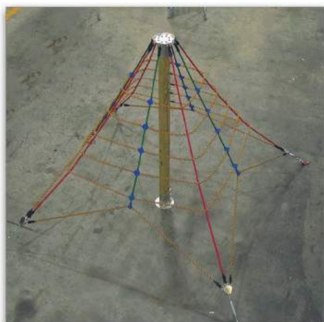
Ref. 299-C Pirámide de Escalada Climbing Pyramid / Escalade Piramide 2596 x 3280 x 2865
